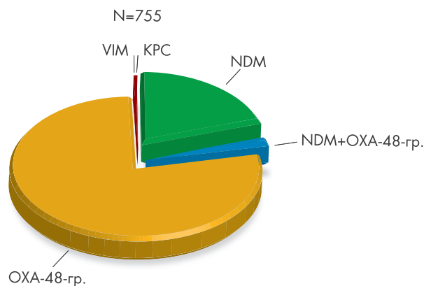
Рисунок 1. Карбапенемазы нозокомиальных штаммов Enterobacterales на территории РФ (2010-2016 гг.)
