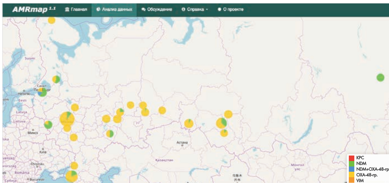
Рисунок 2. Географическое распространение различных типов карбапенемаз среди энтеробактерий в РФ
