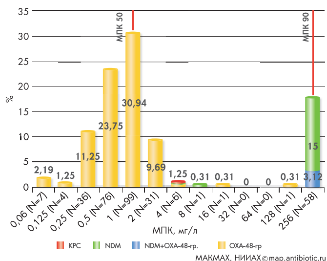
Рисунок 3. Значения МПК цефтазида-авибактама в отношении Enterobacteriales (n=320) с известными типами карбапенемаз
